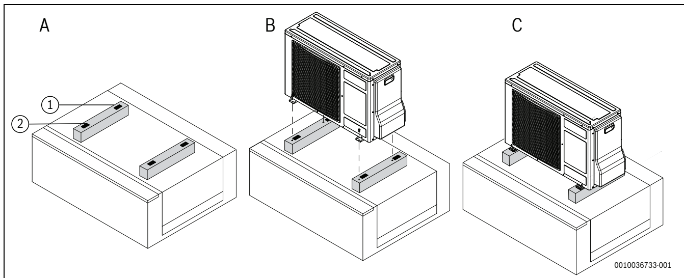
Afb. 9 Vloerstaande buitenunit
