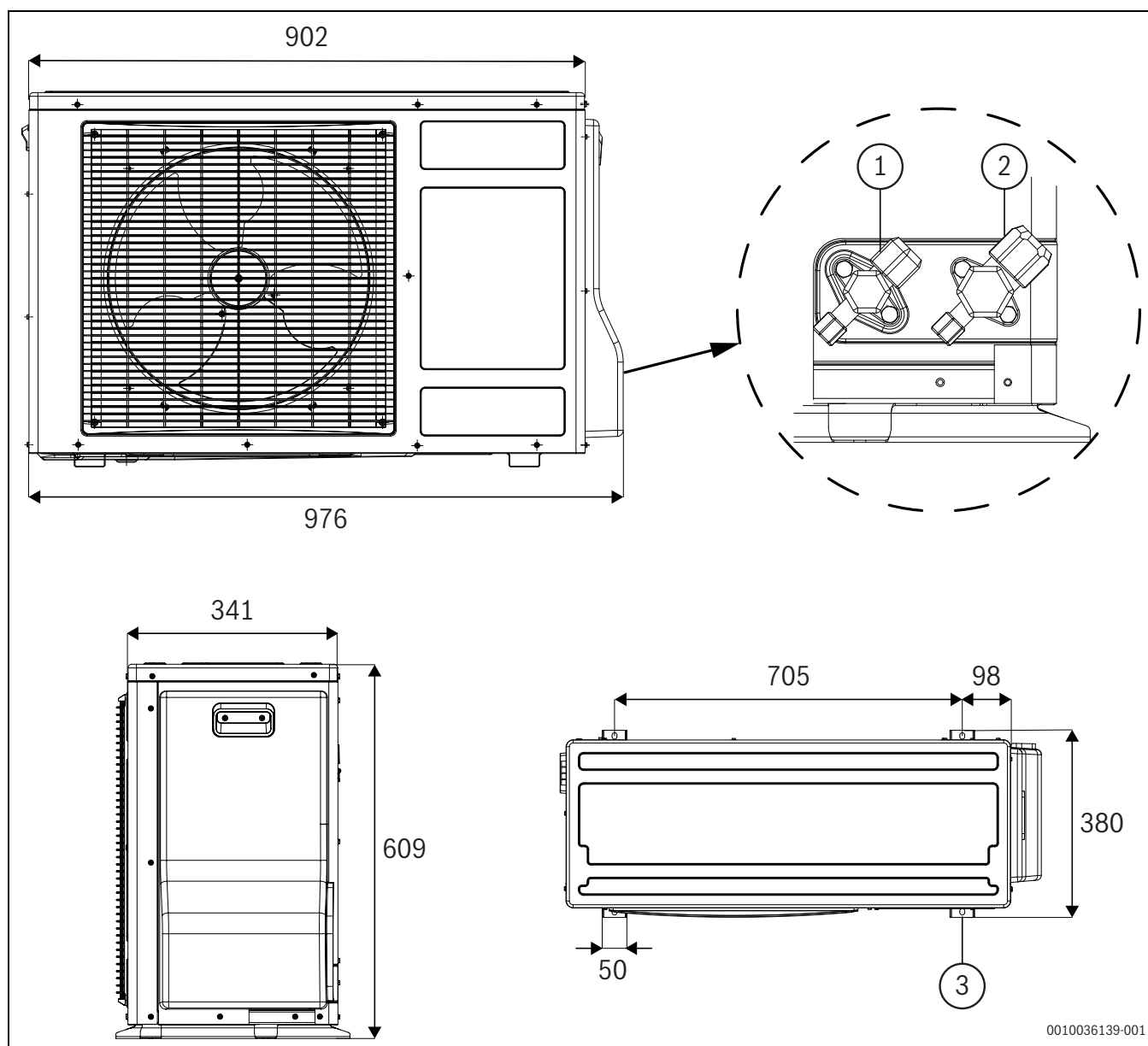
Afb. 2 Afmetingen van de buiteneenheid CS3400iAWS 4 OR-S
