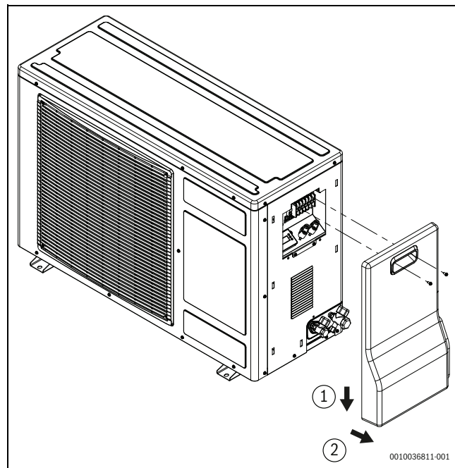
Afb. 14 Verwijder de zijafdekking
