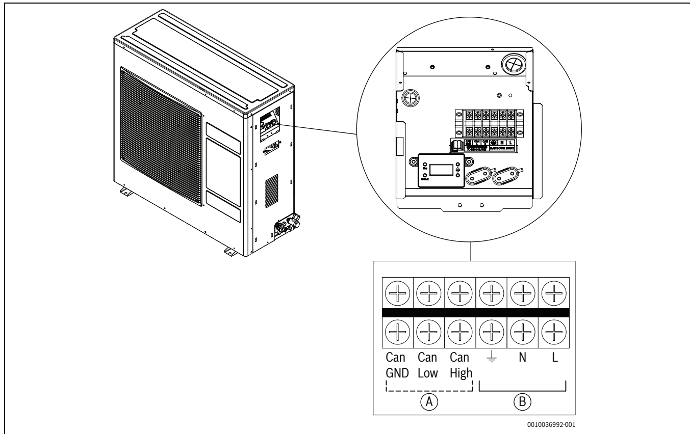
Afb. 19 Kabelaansluitingen
