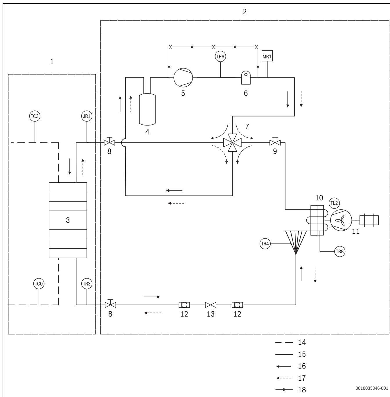
Afb. 25 Diagram koudemiddelcircuit
