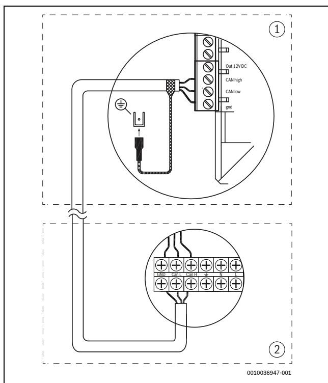
Afb. 20 CAN-BUS-aansluiting
