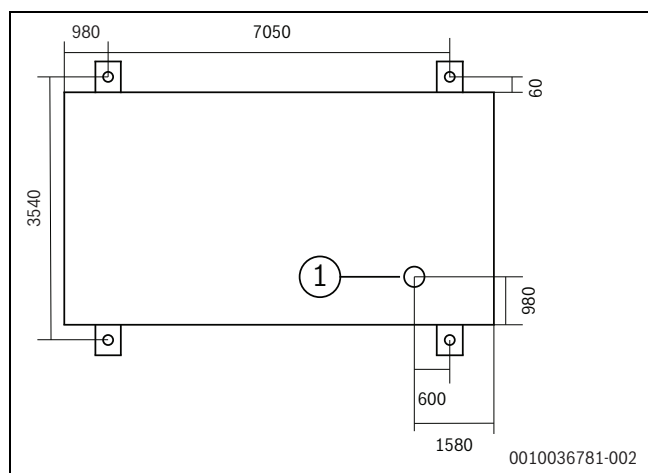
Afb. 7 Bodemplaaf buitenunit (mm)
