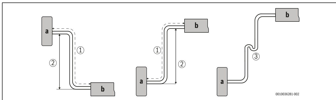
Afb. 10 Leidinglengte en opvoerhoogte
