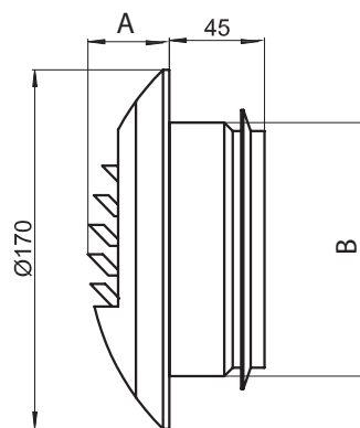
Afbeelding 3.0: Maatschets STR
